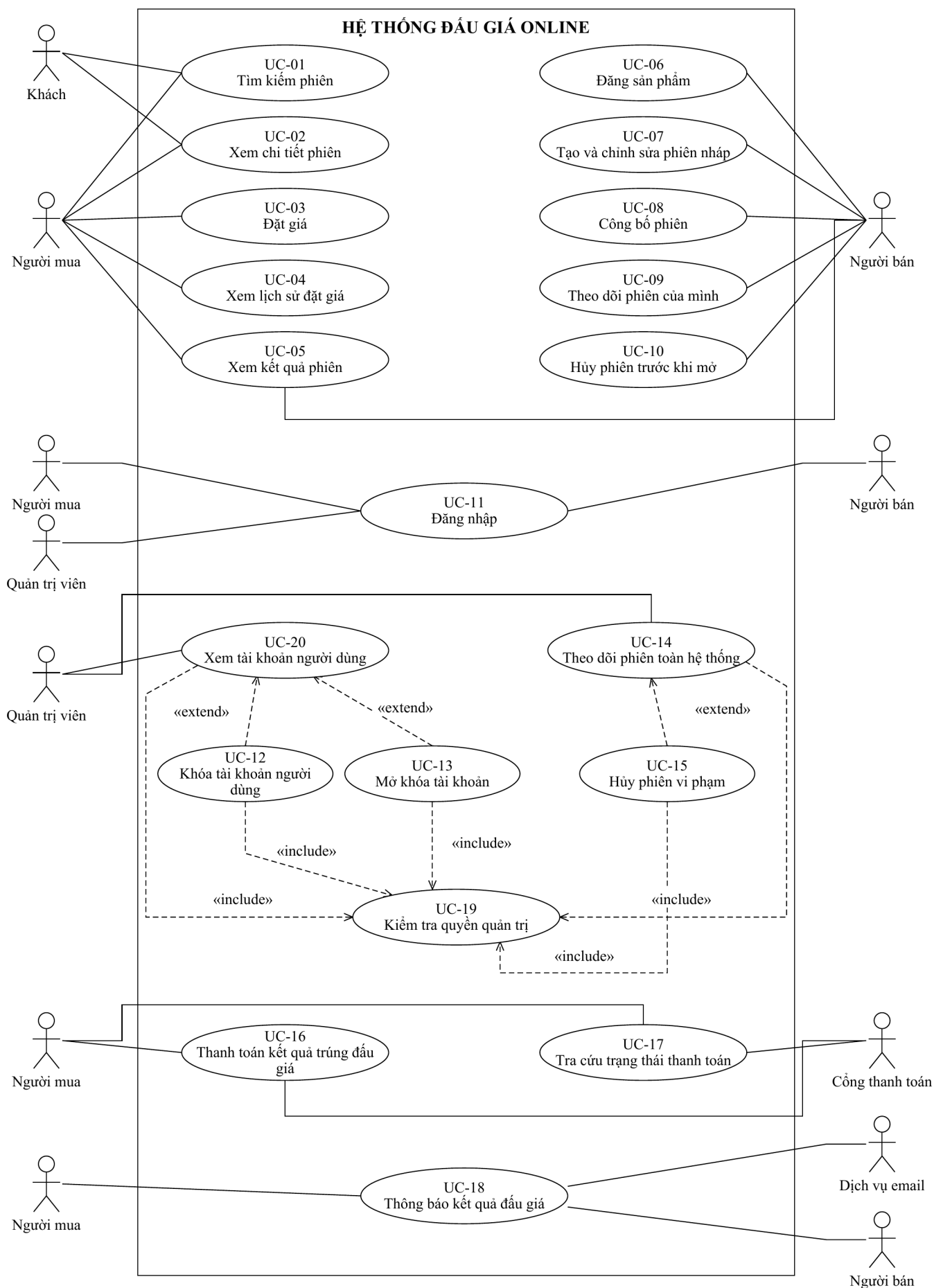
Hình 1. Sơ đồ Use Case; actor lặp cùng tên là cùng một vai trò.
